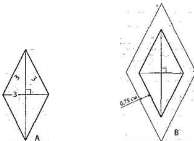
Рис. 55. Шабли ромбів: А — без припусків на шви; В — з припусками на шви.
